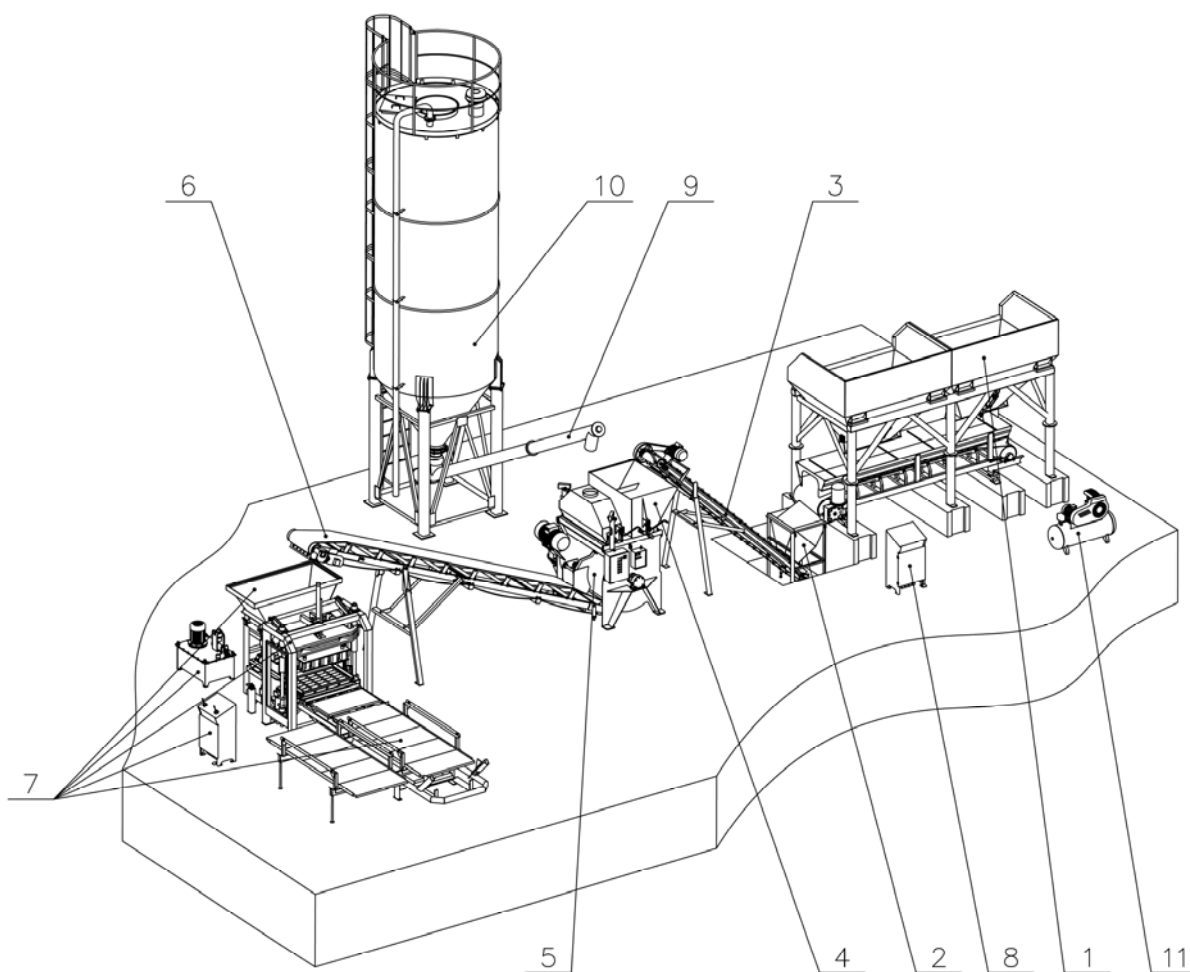
Рис. 1. Общий вид комплекса.
